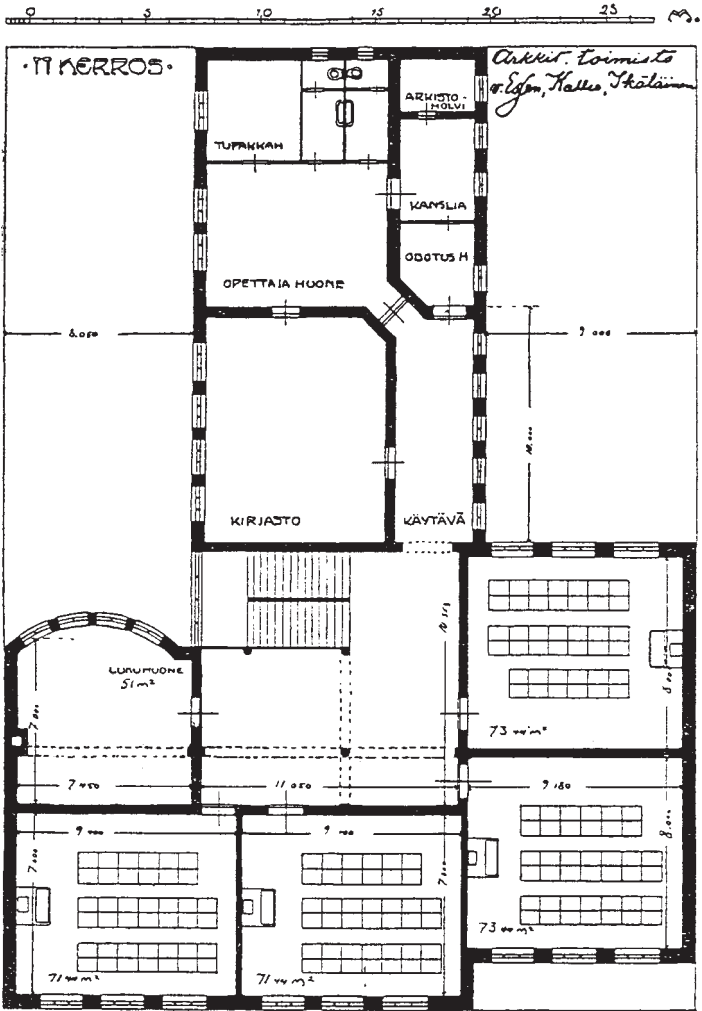
Toisen kerroksen pohjapiirros.
