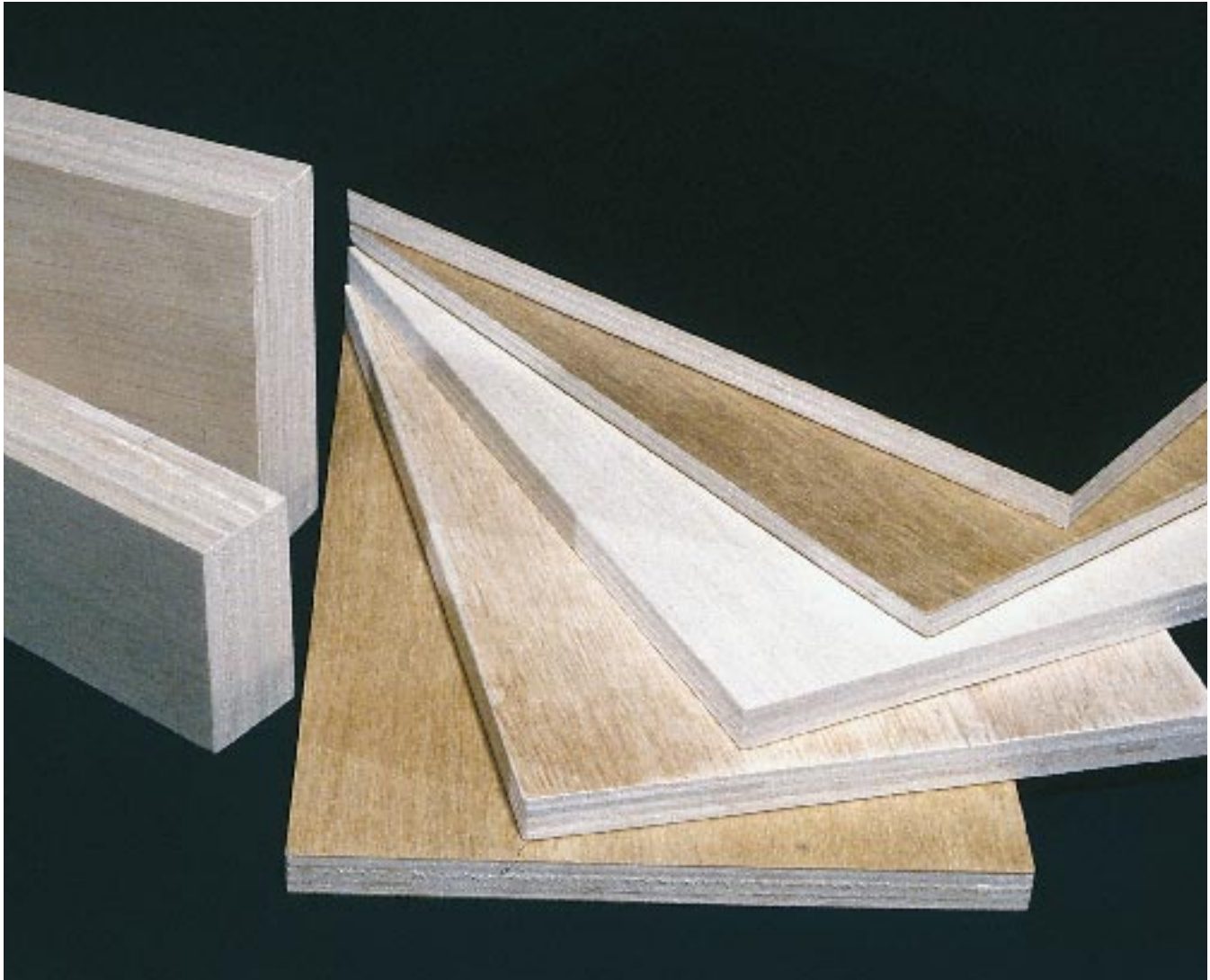
Albizia Falcataria -puusta valmistettuja koelevyjä. Laboratorio-olosuhteissa voidaan valmistaa asiakkaan raaka-aineista lopputuotteita. Näin varmistetaan puun soveltuvuus tuotannolliseen käyttöön ennen investointipäätöksen tekoa.
