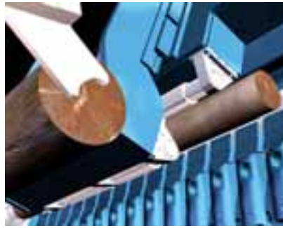
Vahvan tuotekehityksen tuloksena syntyneet pitkälle automatisoidut sorvauslinjat parantavat asiakkaan kilpailukykyä.
